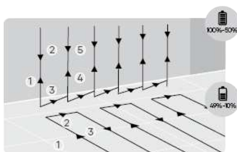
Modo de limpieza automática: limpieza de fondo y paredes de la piscina
