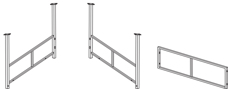
Left side frame Cadre latéral gauche Ax1
